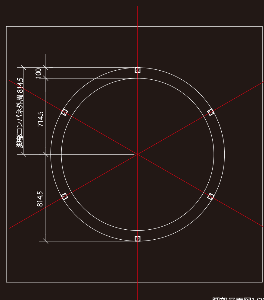
脚部平面図1/20
