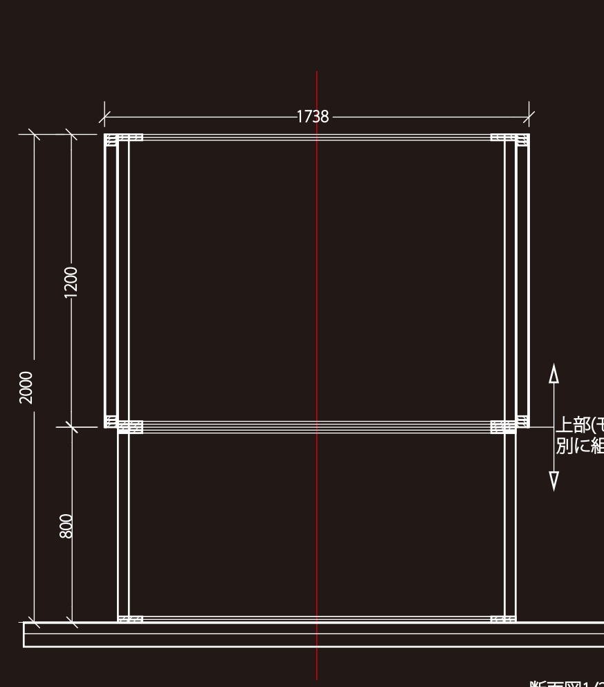
断面図1/20
