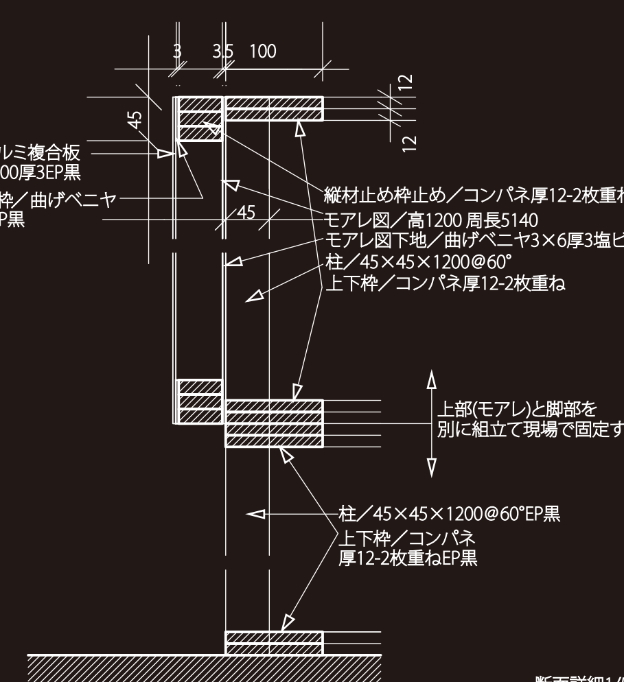
断面詳細1/5
