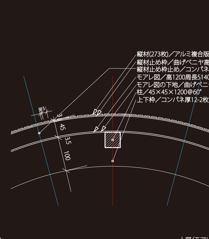
上部(モアレ) 平面詳細1/5
