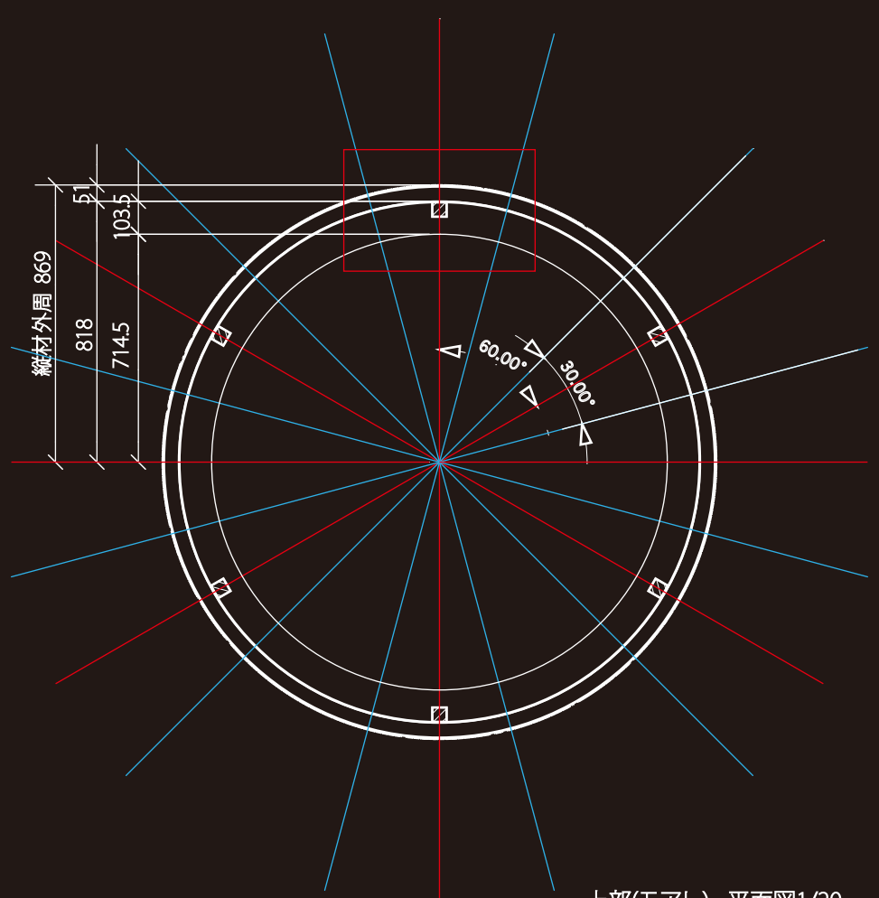
上部(モアレ) 平面図1/20
